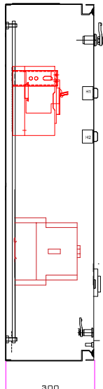
VISTA LATERAL
